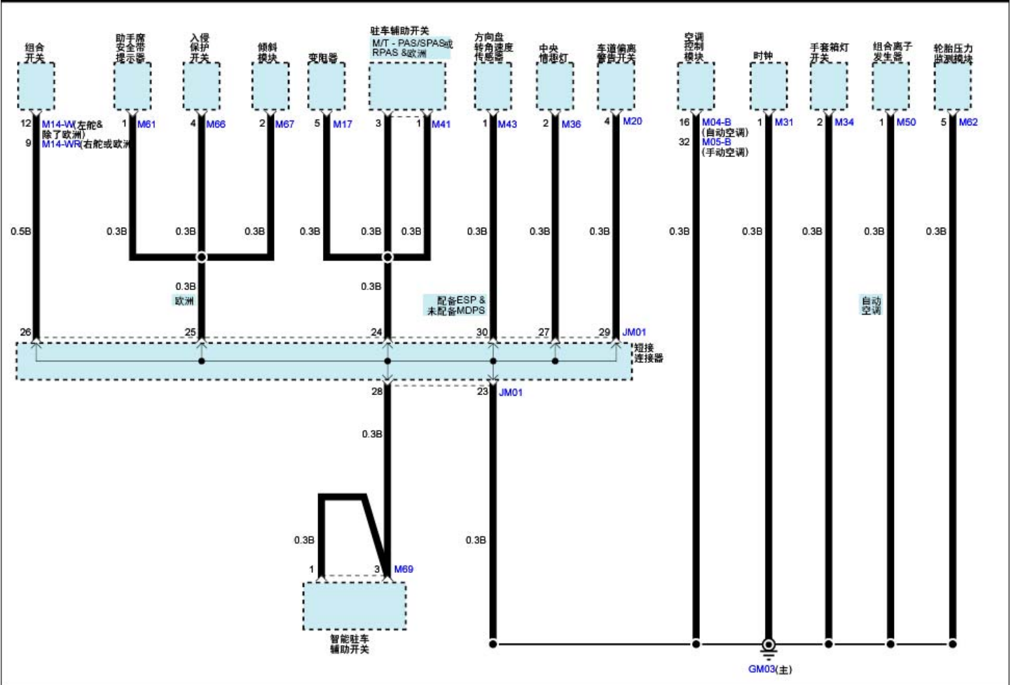
搭铁分布(3)
